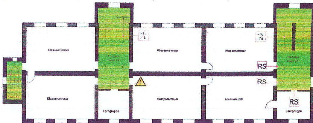
Helbra Grundschule Hauptgebäude: EG
