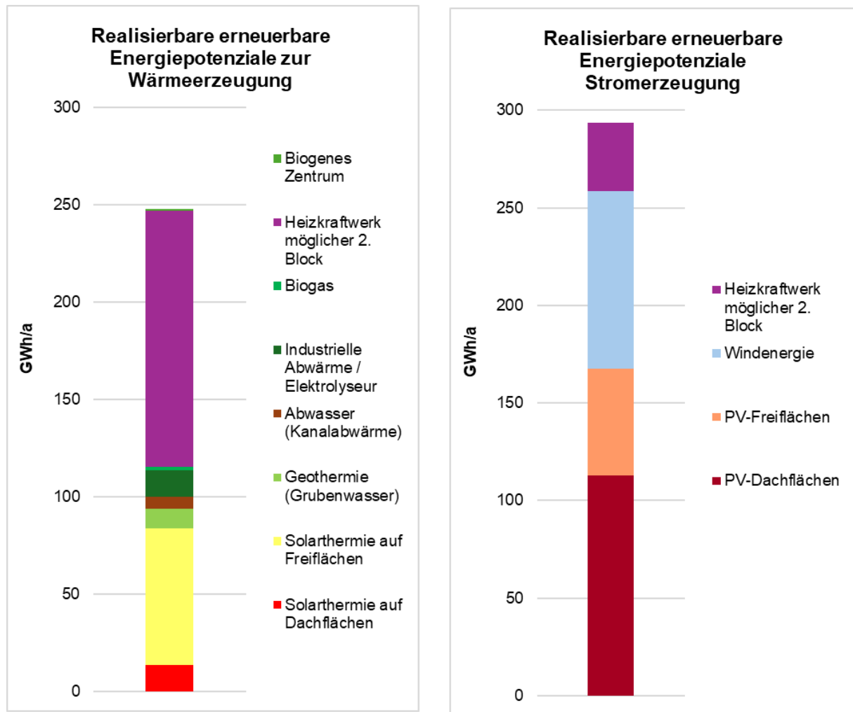
Abbildung 44: Zusammenfassung der Potenziale erneuerbarer Energien
